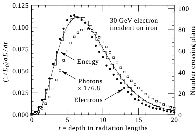
Рис. 14. Продольное развитие ливня, инициированного электроном с энергией 30 ГэВ в железе. Результат моделирования с помощью программы EGS4 [1, 26]. Гистограмма показывает распределение энерговыделения; точки и квадраты представляют числа электронов и фотонов, соответственно, с энергией превышающей 1.5 МэВ; сплошная линия соответствует аппроксимации, данной (46)
