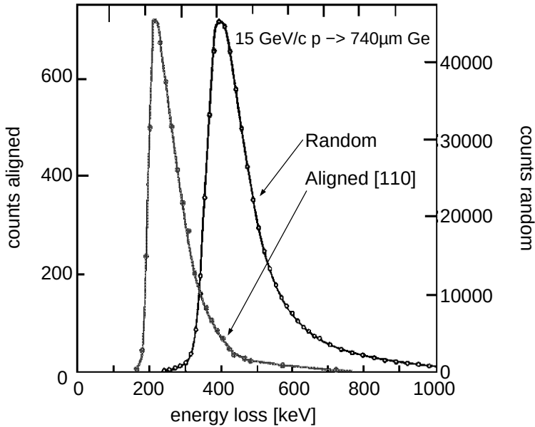
Рис. 4. Потери энергии протонов с энергией 15 ГэВ, проходящих через кристалл германия толщиной 740 мкм [15]
